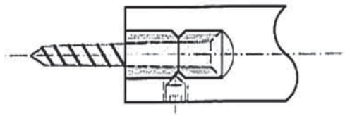
Befestigung für Papier-Rollenhalter, Handtuchhacken, Glasablage, Badetuchhalter, Wannengriff
