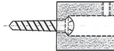
Befestigung für Spiegelhalter
