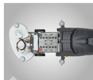
Bürstenköpfe austauschbar, dadurch nur eine Maschine mit unterschiedlichen Bürstenköpfen verwendbar statt verschiedene Maschinen
