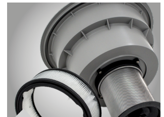
• Doppelfiltersystem für gleichzeitige Nass-/Trockenabholung
