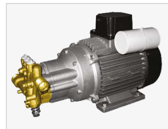
Elektrische Drei-Kolben-Axialpumpe mit Messingkopf Induktionsmotor mit Motorschutzschalter
