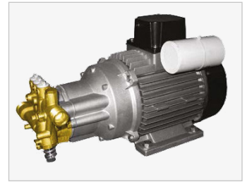
Elektrische Drei-Kolben-Axialpumpe mit Messingkopf Induktionsmotor mit Motoschutzschalter
