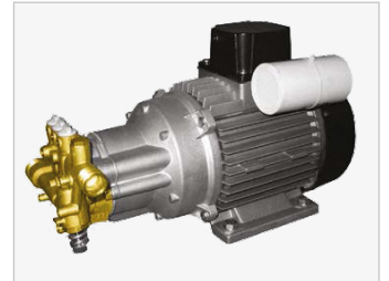
Elektrische Drei-Kolben-Axialpumpe mit Messingkopf Induktionsmotor mit Motorschutzschalter
