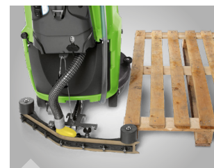
Automatisches Aushaken der Absaugleiste bei unbeabsichtigten Stößen schützt vor Beschädigung
