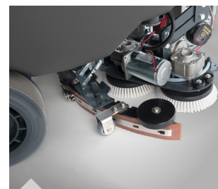
Vier kleine Scheibenbürsten, mit direkt dahinter liegender Absaugleiste, ermöglichen eine kurze Bauform und einen sehr kleinen Wendekreis.
